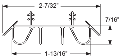
Tru-Defense Door Bottom Sweep
