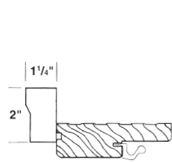
908 Brickmould
